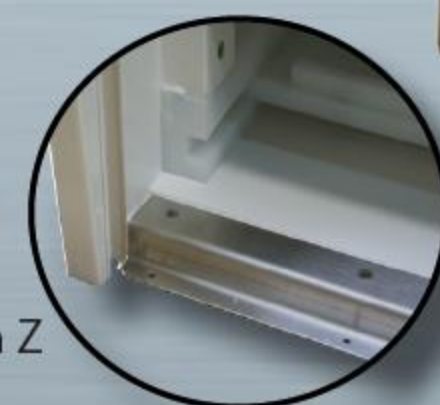
AGRO PM avec option PM 401
